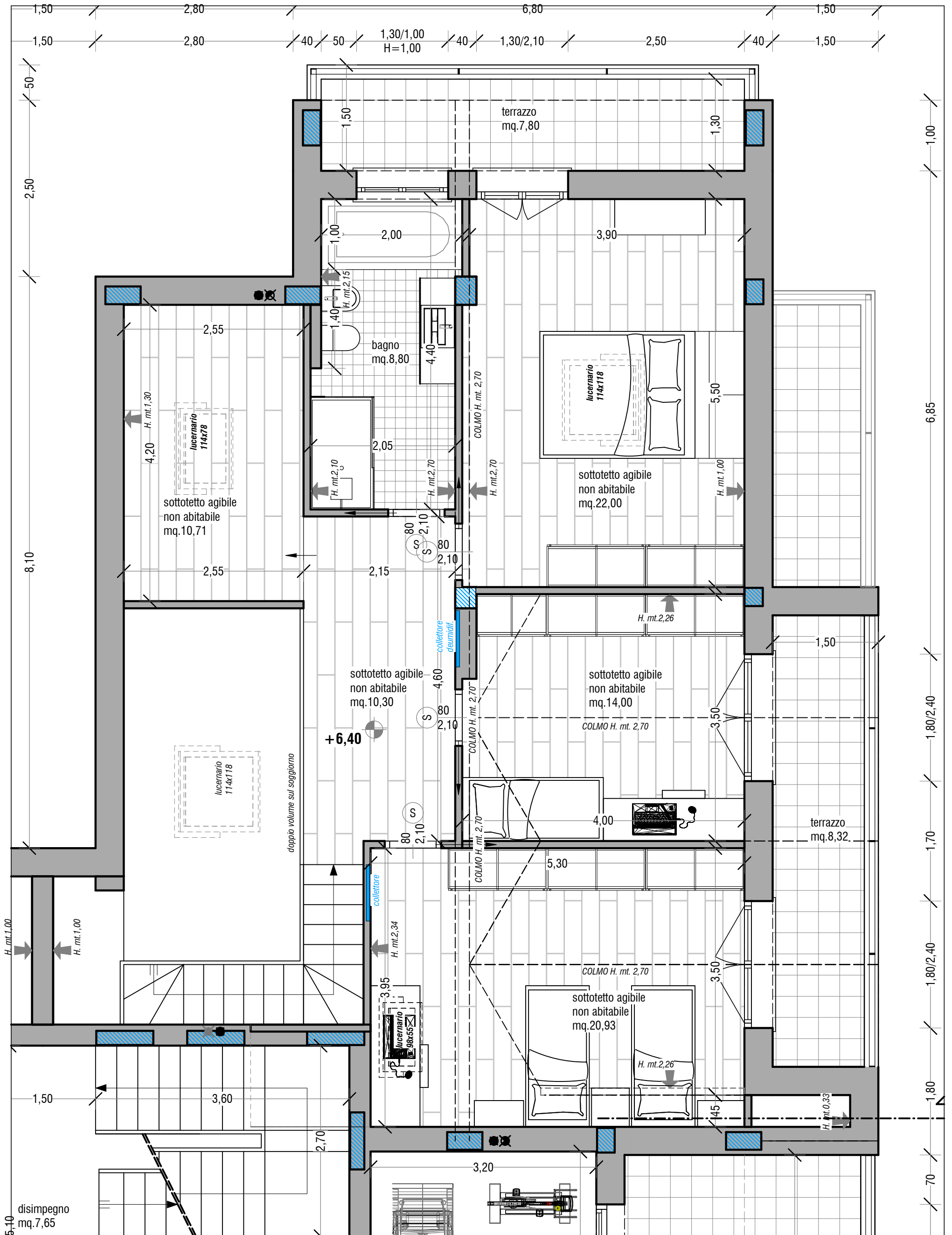
TREVIGLIO (BG) via Bressana - A.Vi.Bi. Immobiliare S.r.l. PIANO SOTTOTETTO - Appartamento 5 - scala 1:50
